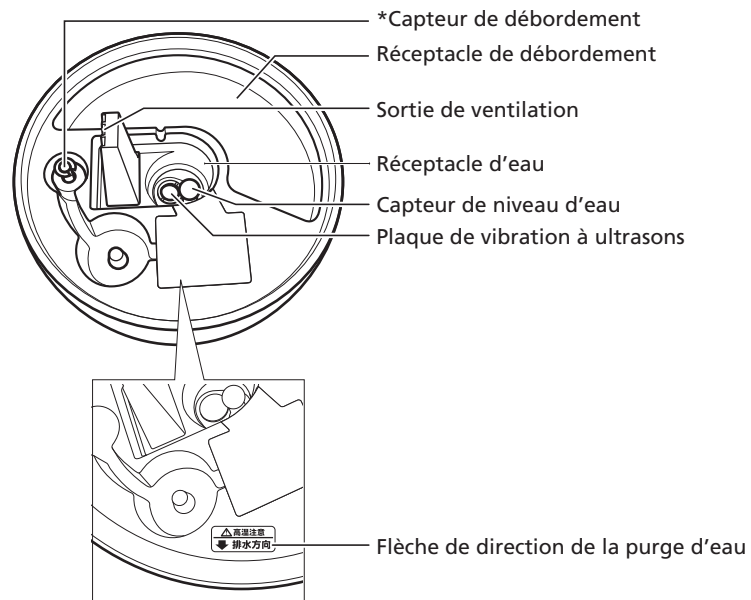
Face arrière du réservoir d'eau
